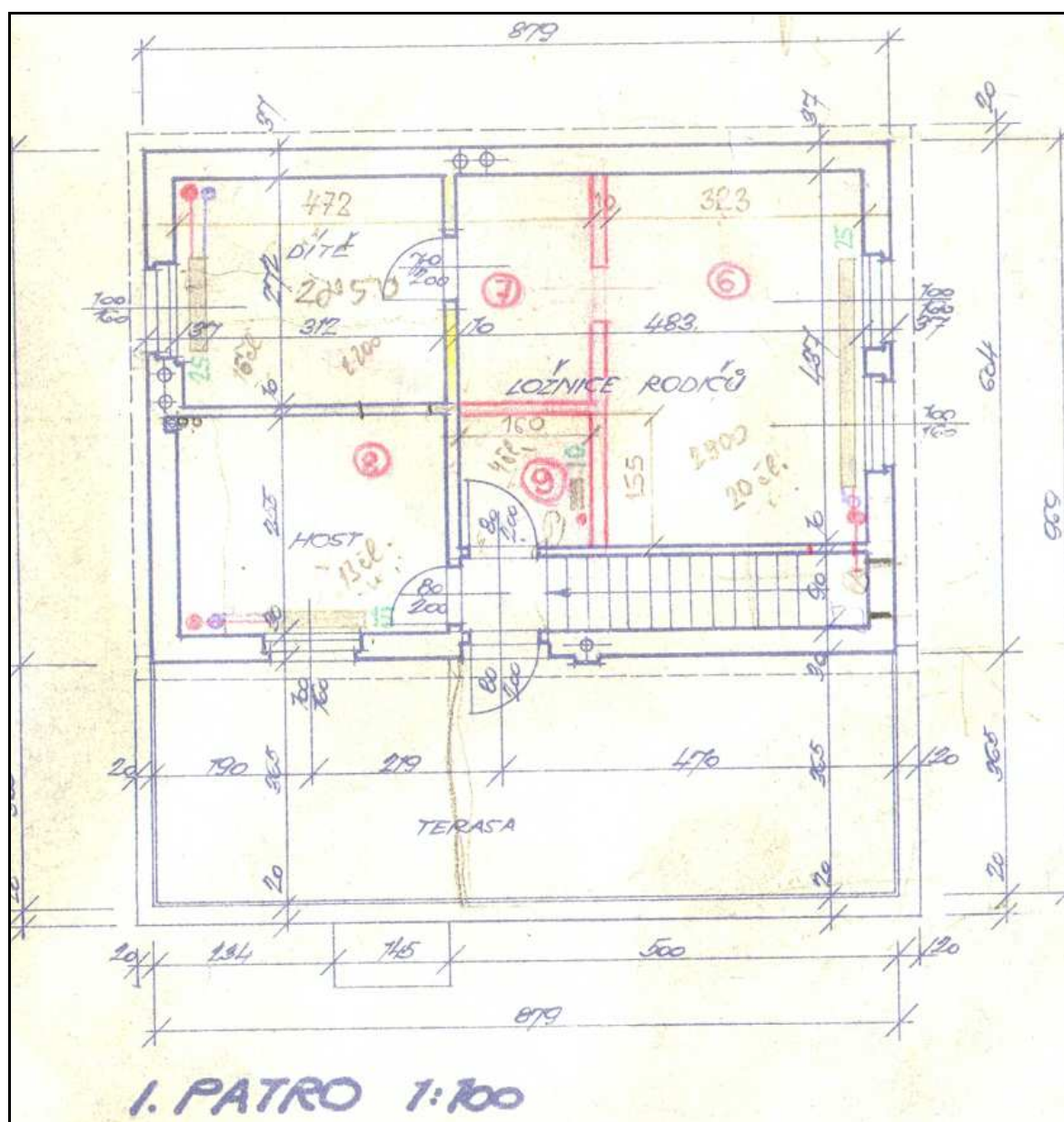
Kopie původního plánu ke stavbě – I. patro
